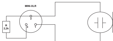
Condensatore senza resistore interno di pull-up.
