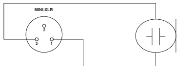
Condensateur avec résistance d'excursion interne.
