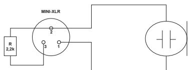
Kondensator bez wewnętrznego rezystora podciągającego.
