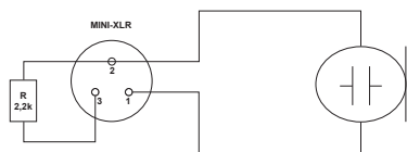
Condensador sin resistencia interna.
