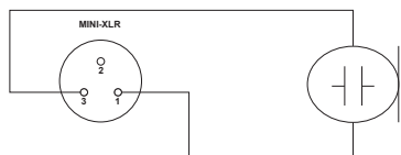
Condensador con resistencia interna.
